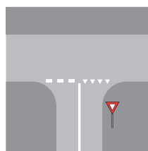
6.16.1 Linea di guida dopo una linea d'attesa (art. 76)
